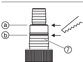
Schlauchverbindung des Universal-Anschlusses (7)
