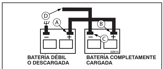
Fig. 44
