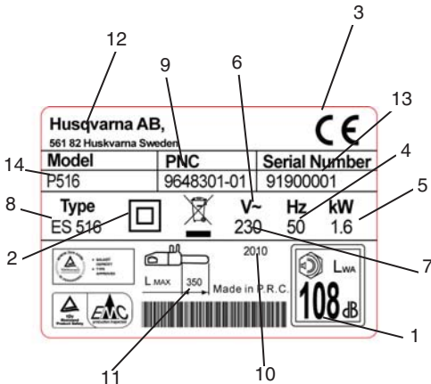
Exempel på märkplåt
