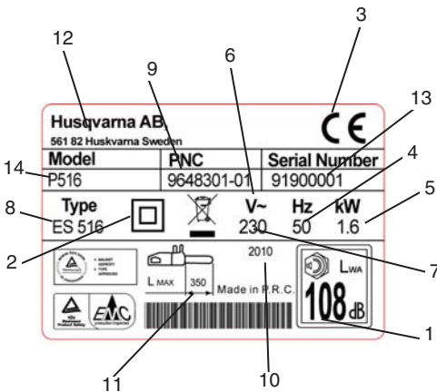
Exemplu de etichetă pentru identificare
