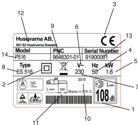
Primjer naljepnice s podacima
