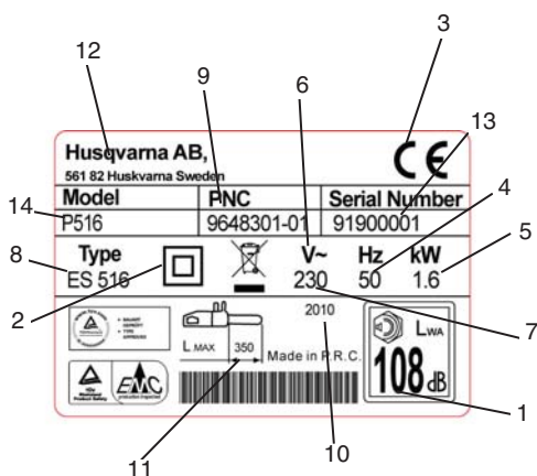
Ražotāja etiķetes piemērs
