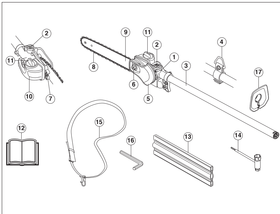
Imena delov nastavkov žage. (Prikluček za žaganje z držalom PA 1100)
