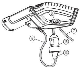
Pripojenie nožnic na živý plot:
