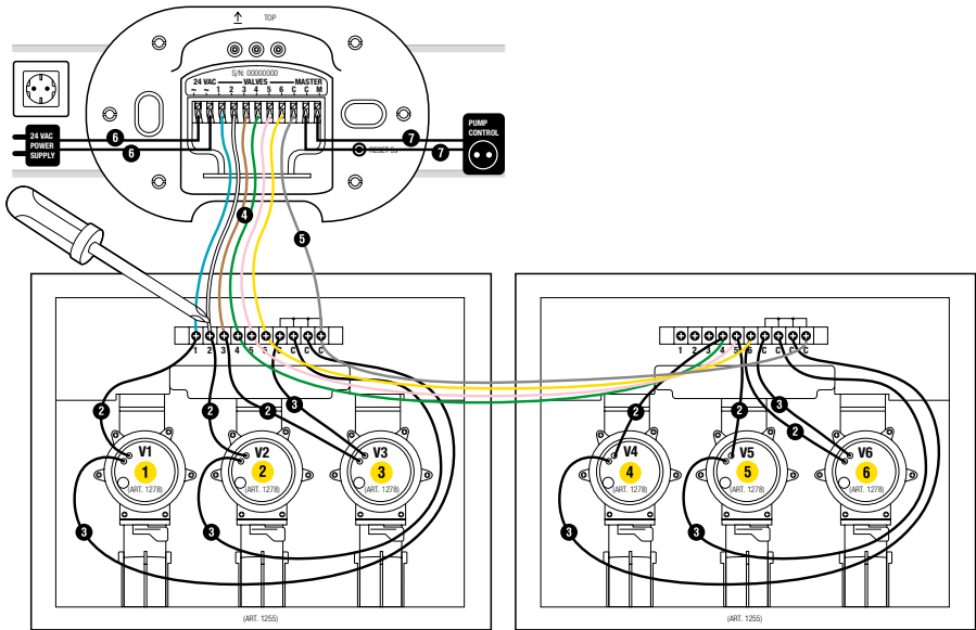
Ventielbox art. 1255
