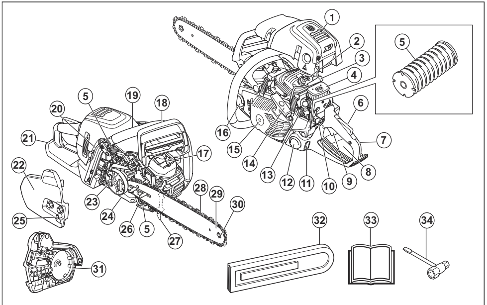
1. Кришка циліндра
