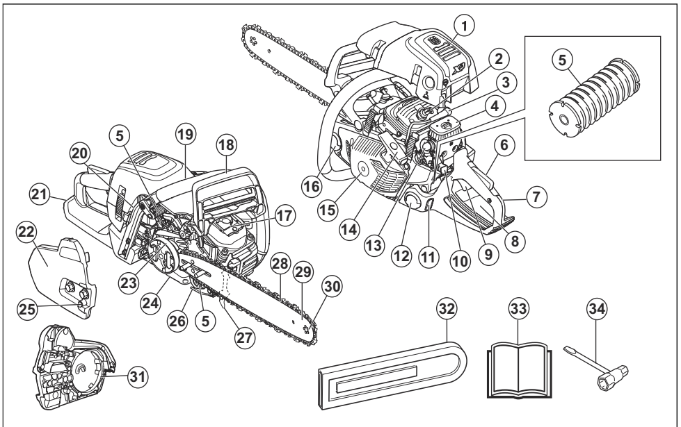
1. Крышка цилиндра
