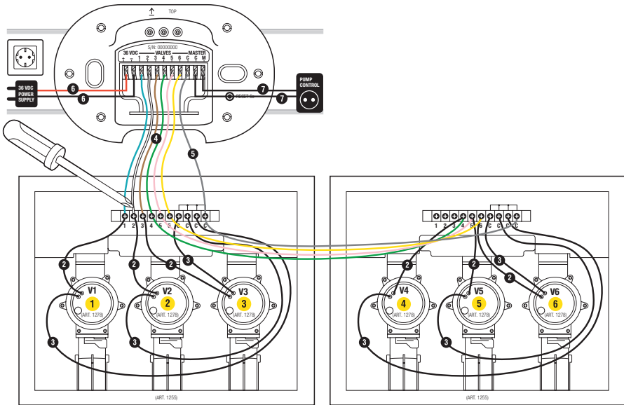
Caixa de válvulas, n.º de ref. a 1255 Caixa de válvulas, n.º de ref. a 1255
