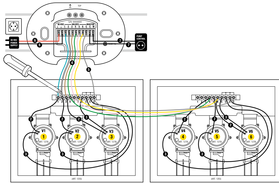
Ventielbox art. 1255
